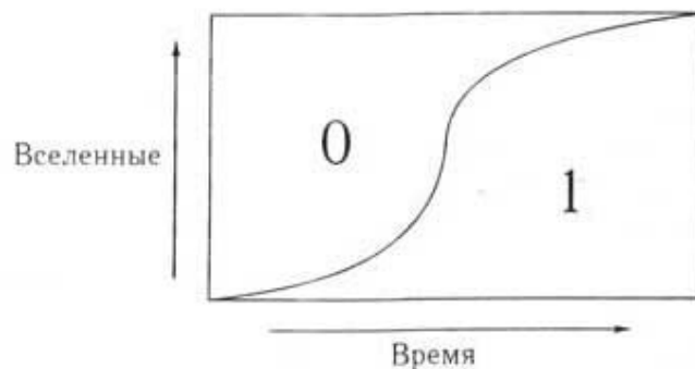
Рис. 9.4. Перспектива мультиверса на непрерывное изменение бита от 0 до
