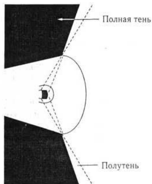
Рис. 2.3. Полная тень и полутень тени
