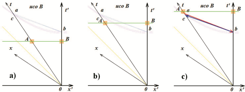
Рис.26.7. Обмен сверхсветовыми сигналами с точки зрения системы В. Приведены кадры из анимации [21] обмена тахионом двумя ИСО А и В.
