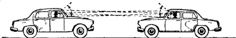
Рис.5.2. Каждому шоферу ветровое стекло своей кабины видно под большим углом зрения, чем такое же стекло встречного автомобиля [98]
