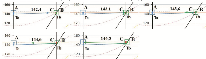
Рис.27.6. Процесс обмена тахионами с точки зрения системы А. Скорости прямого и обратного тахионов равны. На диаграммах они разнесены, чтобы устранить их визуальное слияние. Кадры из анимации [21].
