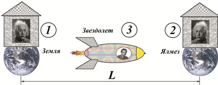
Рис.6.2. Вариант парадокса близнецов – три близнеца
