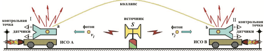
Рис.20.3. Две движущиеся инерциальные системы с точки зрения неподвижной ИСО. Источник запутанных фотонов неподвижен и фотоны из каждой пары приходят в движущиеся ИСО одновременно. Строенные стрелки-молнии указывают на точки, в которых находились фотоны в момент коллапса волновой функции.
