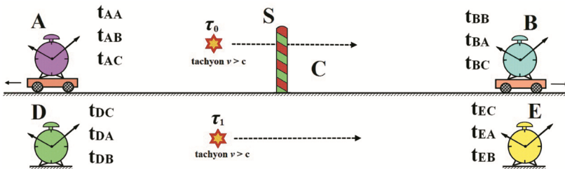
Рис.24.2. Отправленный из А тахион прибедет к В точно в то же, время, что показывают часы А.
