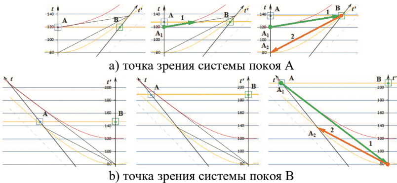
Рис.26.1. Парадокс антiteleфона а) с точки зрения системы покоя, б) с точки зрения системы покоя В. Фрагменты кадров из анимации [21]
