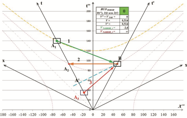
Рис.26.4. Парадокс антiteleфона с точки зрения неподвижной ИСО. По отношению к ней наблюдатели А и В движутся в противоположных направлениях с одинаковой скоростью.
